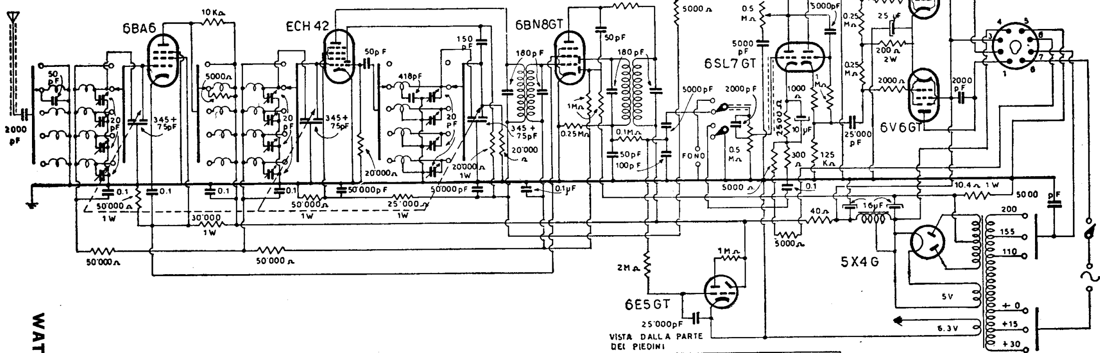
WATT RADIO - Mod. GIUBILEO FONDO - Medie e tre corte. Media frequenza a 470 kc. Tensioni come il mod. Giubileo.
